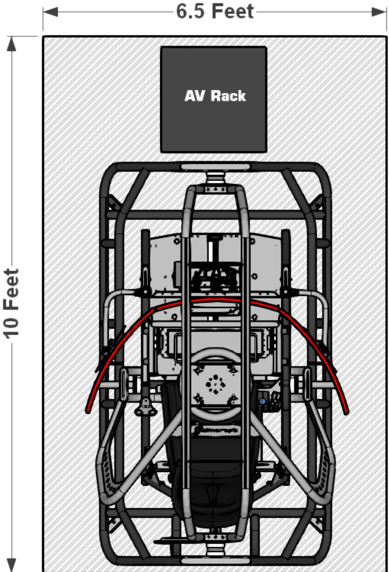
APEX GT | Triple Curved 32" | Front AV Rack Dimensions
