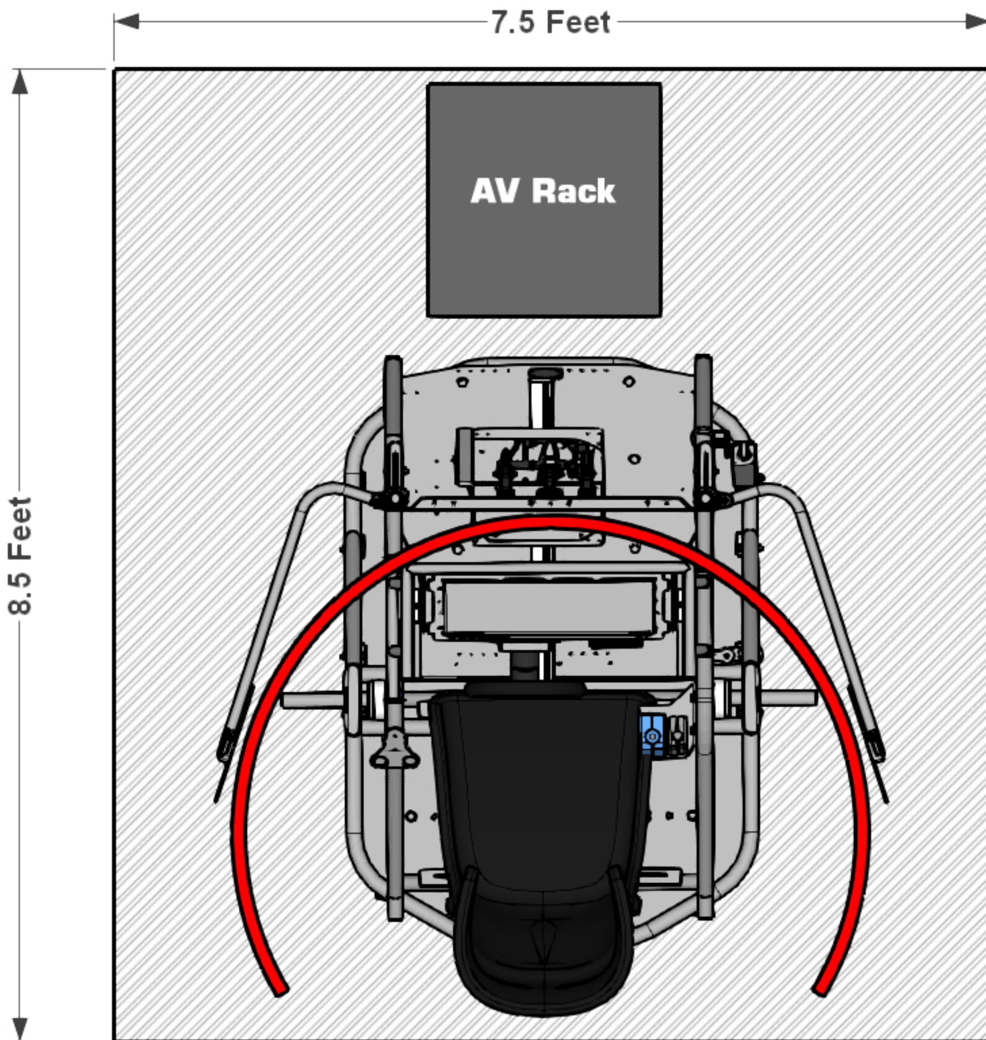
APEX CT | Triple Curved 45" | Front AV Rack Dimensions
