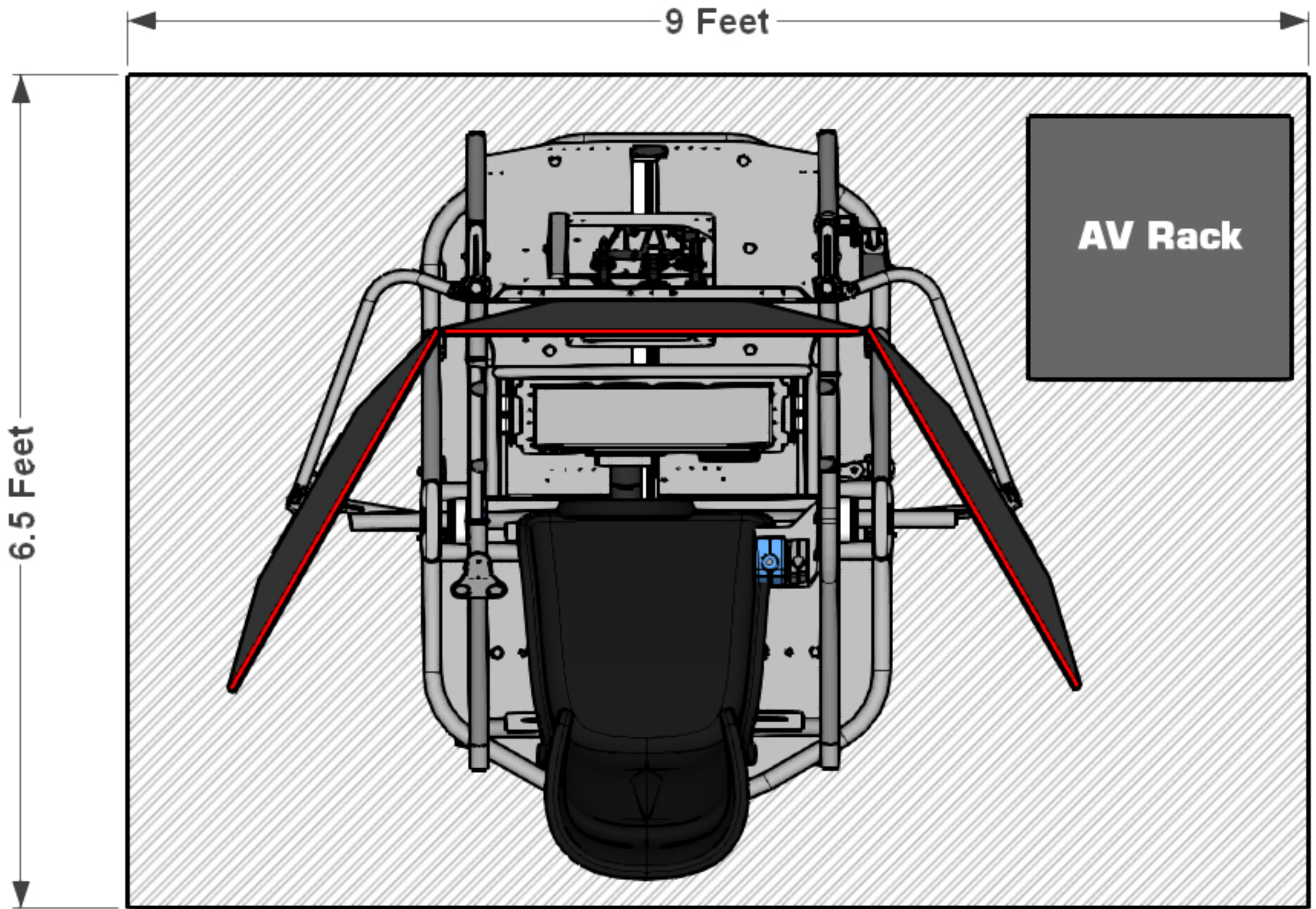
APEX CT | Triple Flat 43" | Side AV Rack Dimensions
